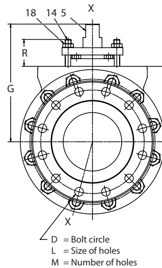
8" (DN 250) Class 150 6" & 8" (DN 150 & 200) Class 300
