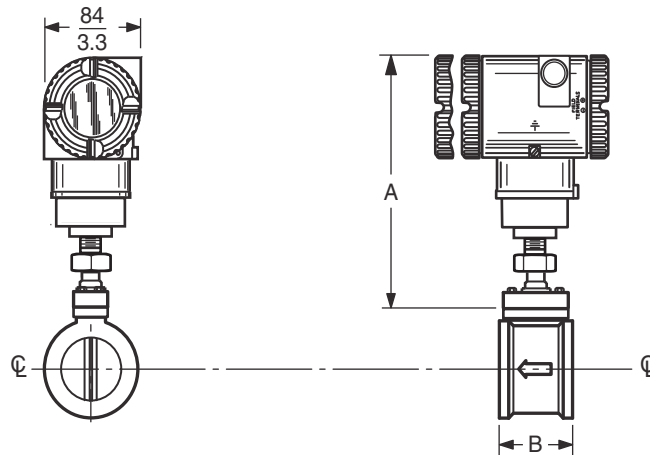
84C WAFER BODY
